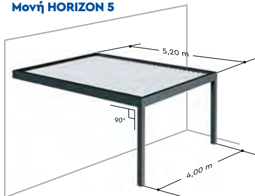
Μονή HORIZON 5
