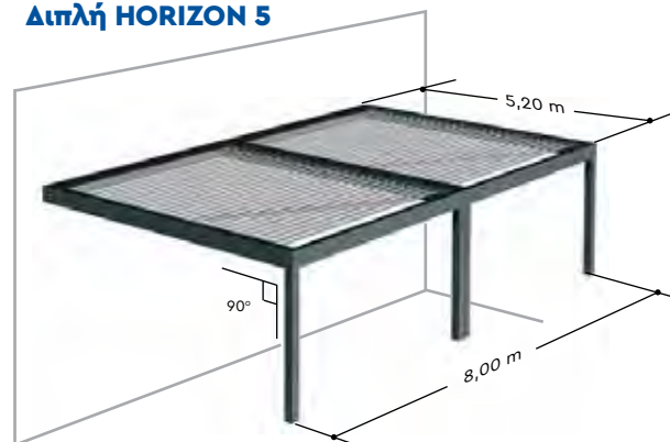
Διπλή HORIZON 5
